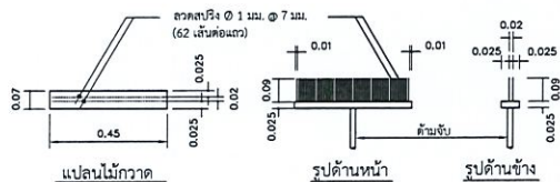
รายละเอียดไม่กวาดผิวหน้า ค.ส.ล. NOT TO SCALE
